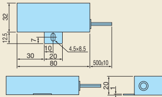
TK50B 30ΩJ (HF5B0416)
