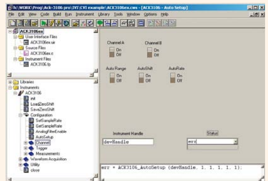
Использование функционального дерева инструмента в LabWindows/CVI
