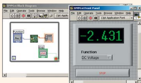
LabVIEW 3 программа цифрового мультиметра
