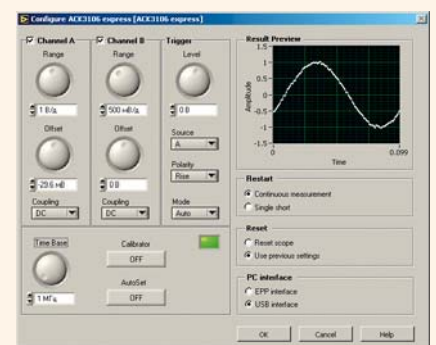
Диалоговая панель настройки экспресс-инструмента АСК-3106
